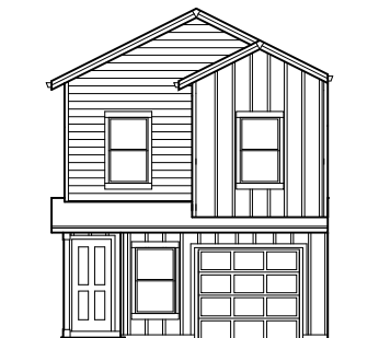
ELEVATION 'W'
